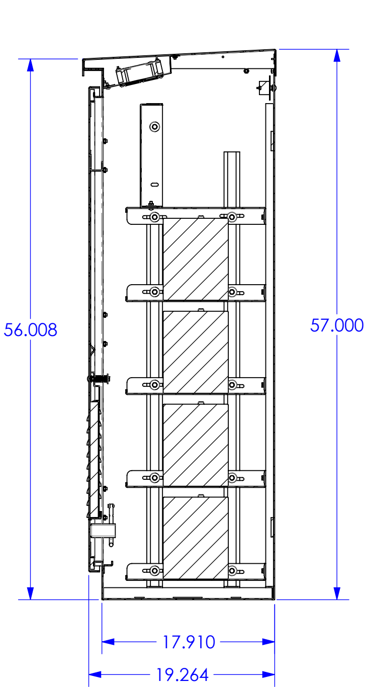
SECTION D-D
